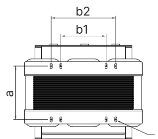
Type2. 175kVA ~ 325kVA
