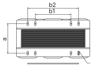
Type1. 112.5kVA ~ 150kVA
