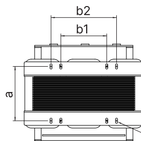
Type2. 175kVA ~ 325kVA
